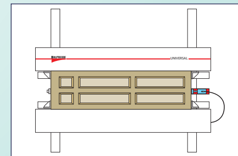
cilindro e riscontro orizzontale supplementare cylinder and relative horizontal fence
